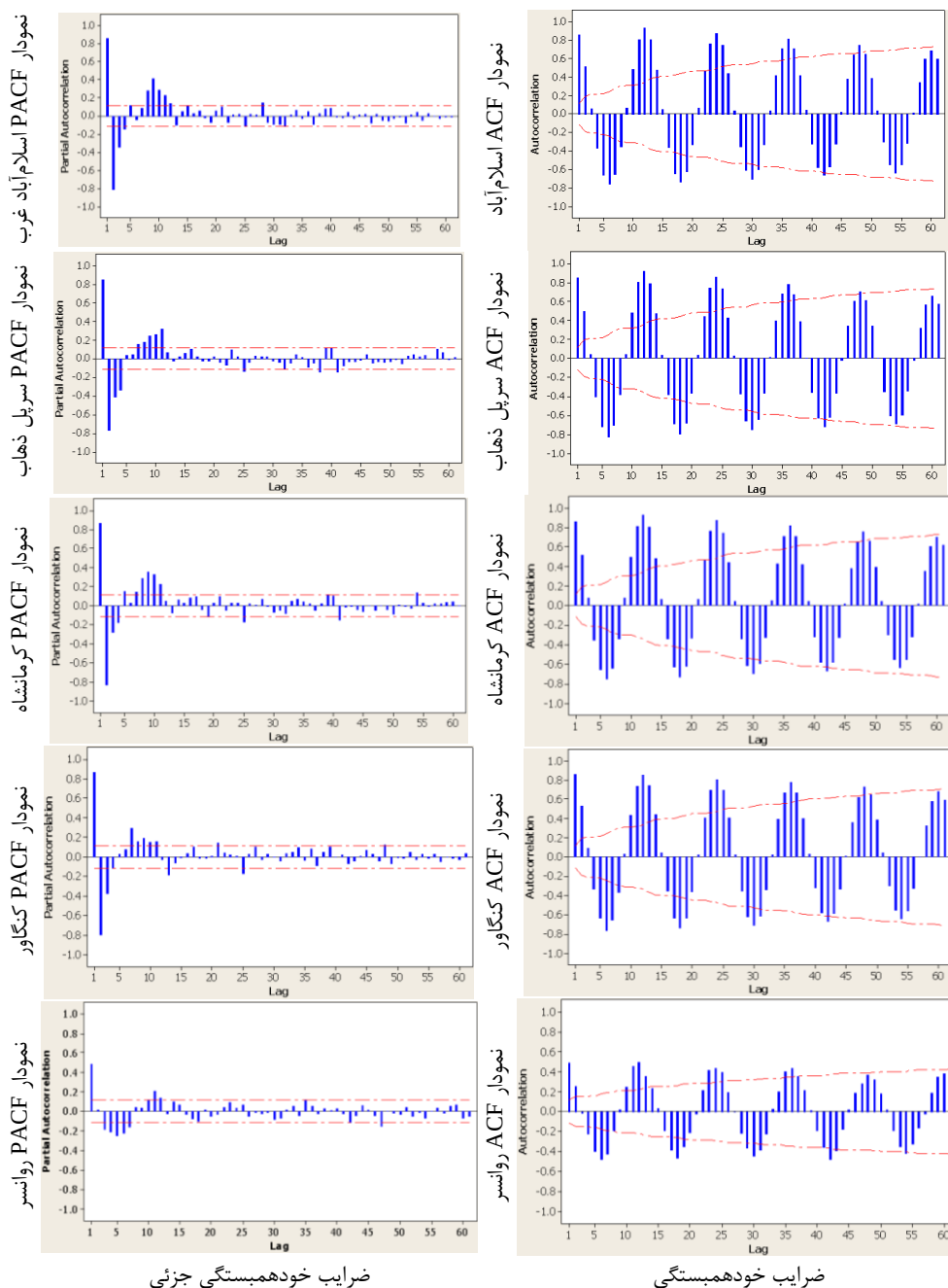
شکل ۳- نمودار خودهمبستگی و خودهمبستگی جزئی سری تفاضلی شده تبخیر-تعلق ماهانه گیاه مرجع
