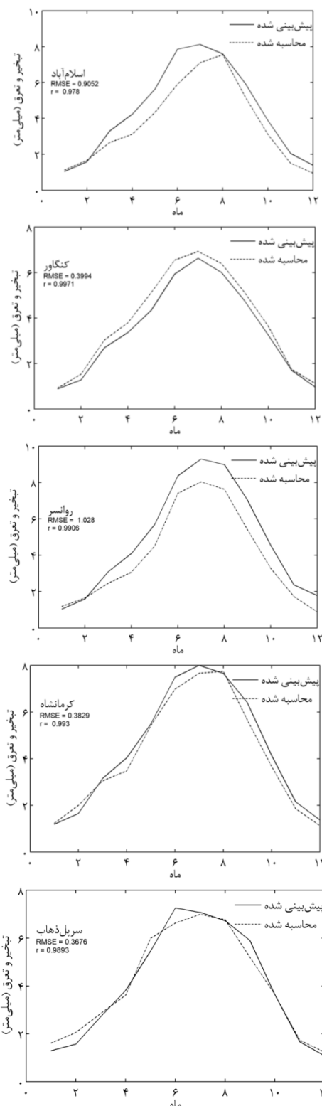
شکل ۵- مقادیر تبخیر- تعرق پتانسیل ماهانه محاسبه شده از رابطه PMF_{56} و پیش‌بینی شده از SARIMA در سال ۲۰۰۹
