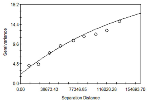
شکل ۳- نیم‌تغییرنمای تجربی و مدل نمایی داده‌های دمای کمینه روز ۲۶ نوامبر ۲۰۰۷
