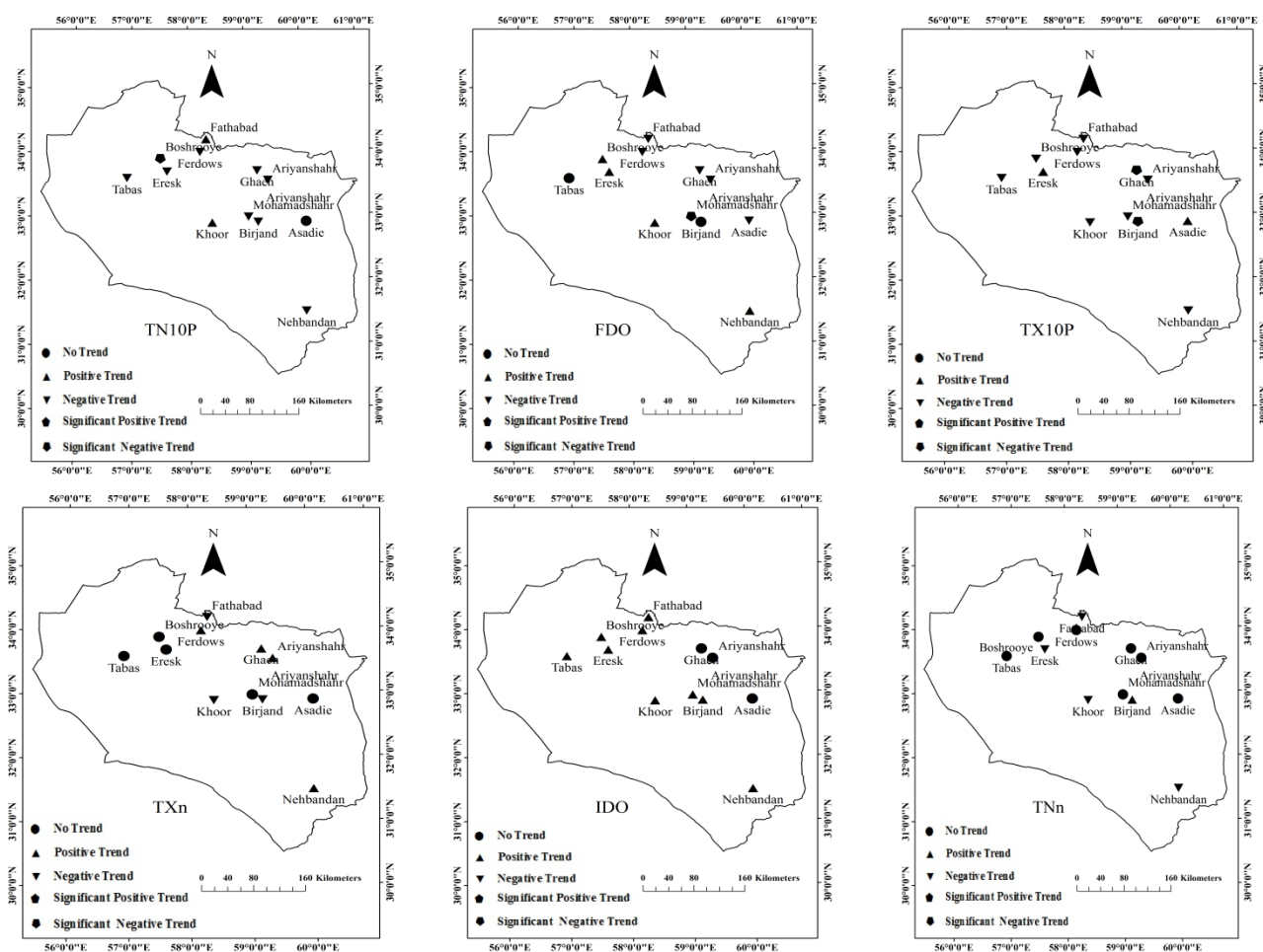
Figure 7- TN10P, FDO, TX10P, TXn, TNn and IDO indices شکل ۷- نمایه‌های TNn, TXn, TX10P, FDO, TN10P, IDO و TNn
